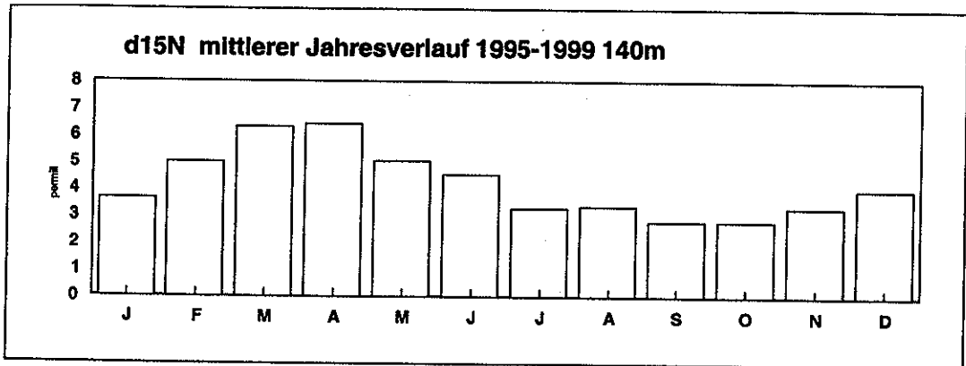
Abb. 14: Isotopie des Stickstoffs (permill delta ^{15}\text{N} ) als Monatsmittel für die Periode 1995-1999.
