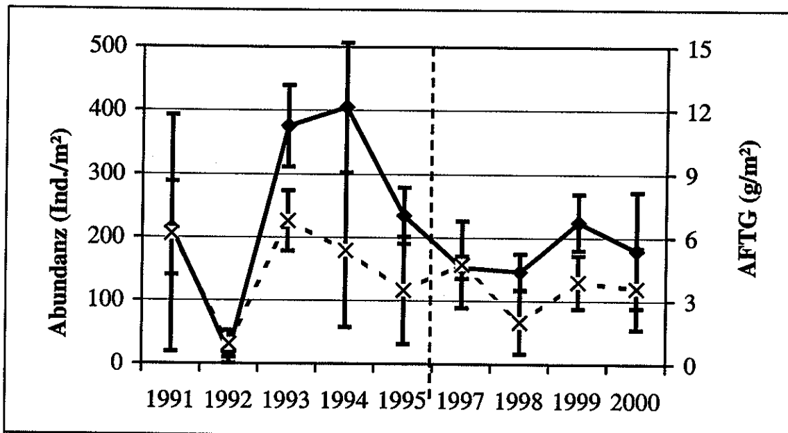
Abb. 34 Entwicklung von Abundanz (♦) und Biomasse (x) von Astarte borealis an der Station 30 von 1991 bis 2000 (1996 keine Daten)
