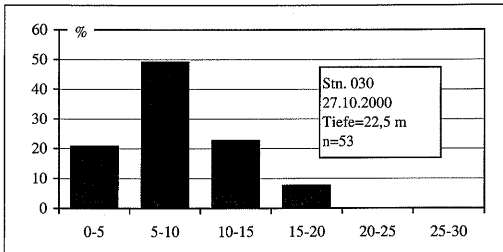
Abb. 35 Größenklassenverteilung von Astarte borealis an Station 30 im Oktober 2000
