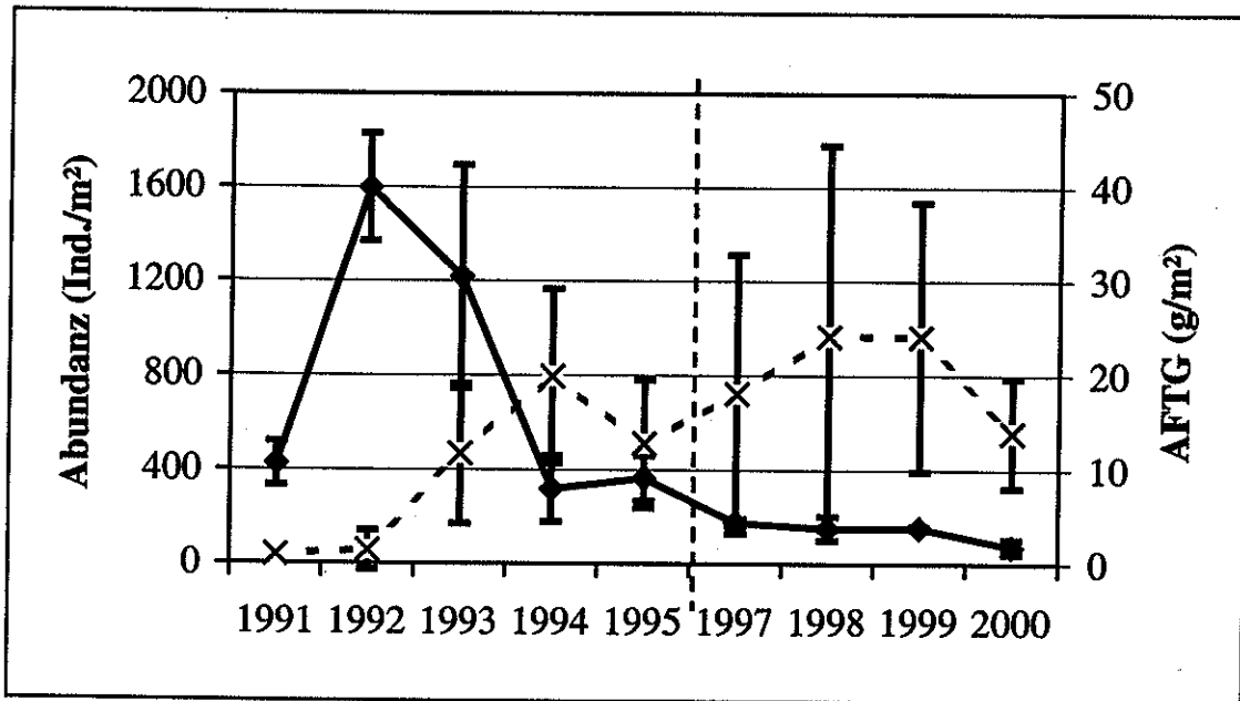
Abb. 33 Entwicklung von Abundanz (♦) und Biomasse (x) von Mya arenaria an der Station 30 von 1991 bis 2000 (1996 keine Daten)
